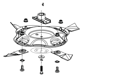
Lâmina Quadcut® LÂMINA TRITURADORA.
