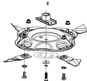
Nóż Quadcut®
