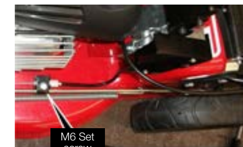
M6 Set screw
