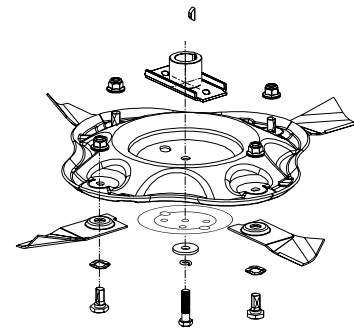
Greito pjovimo geležtė
